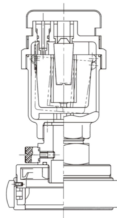
消火栓用空気弁(MV-AV-F)
